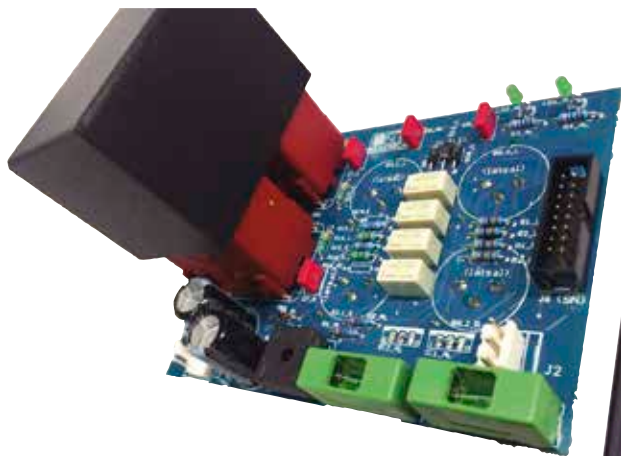
▲ Die symmetrischen Eingänge nutzen zusätzlich gekapselte, hochkarätige Audio-Übertrager.
