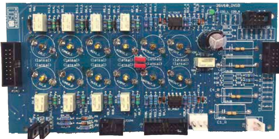
▲ Hier sehen wir die Platine für die (inklusive Masse) relaisgeschalteten, unsymmetrischen Eingänge.
